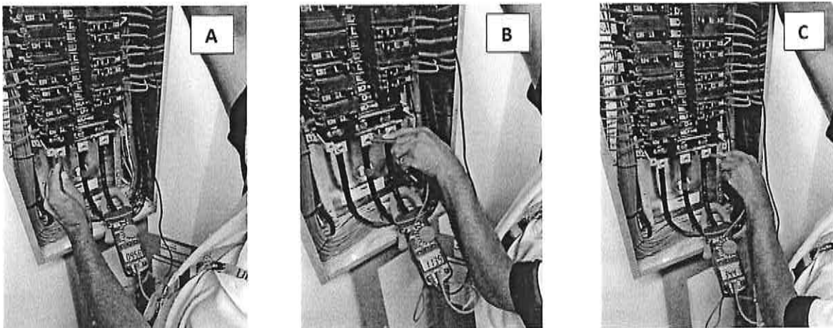
Figura 4 Mediciones de Voltaje en tableros eléctricos. Los valores medidos son los mismos mostrados en la tabla 1
