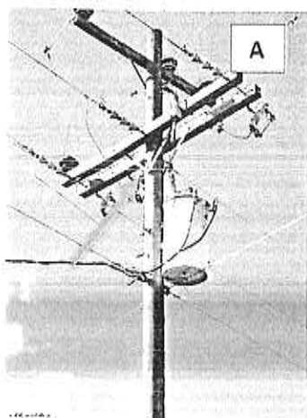
Figura 1.A En la imagen muestra el banco de transformadores de 50 Kva dañado. En la imagen también se señala el portafusible con su respectivo fusible fuera de servicio esto debido a que al existir un falla en el sistema este desconecta el mismo por protección 1.B Debido a que el transformador se encuentra fuera de servicio el edificio de biblioteca no cuenta con energía eléctrica.
