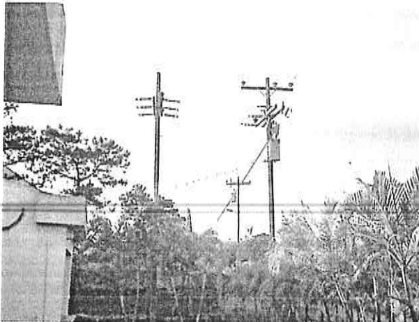
Figura 6. En las imágenes se muestra el tramo de línea primaria que está provocando las fallas en los edificios mencionados en este informe. En la primera imagen se marca el otro posible portafusible dañado.
