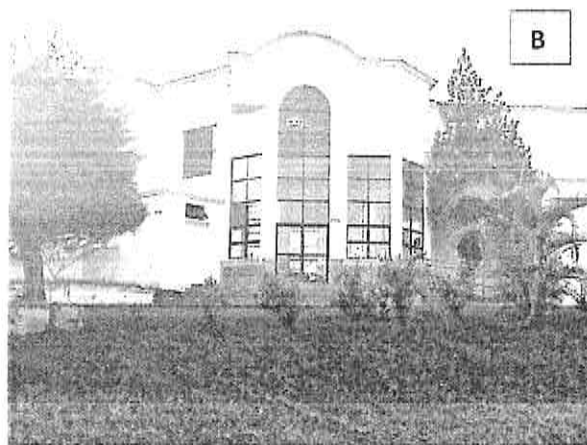
Figura 1.A En la imagen muestra el banco de transformadores de 50 Kva dañado. En la imagen también se señala el portafusible con su respectivo fusible fuera de servicio esto debido a que al existir un falla en el sistema este desconecta el mismo por protección 1.B Debido a que el transformador se encuentra fuera de servicio el edificio de biblioteca no cuenta con energía eléctrica.
